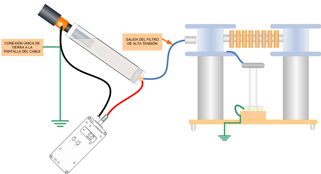
Figura 3. Esquema de conexiones para el calibrador
