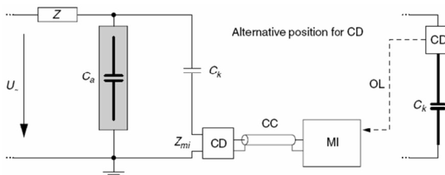
Figura 1. Dispositivo de acople en serie con el capacitor de conexión
