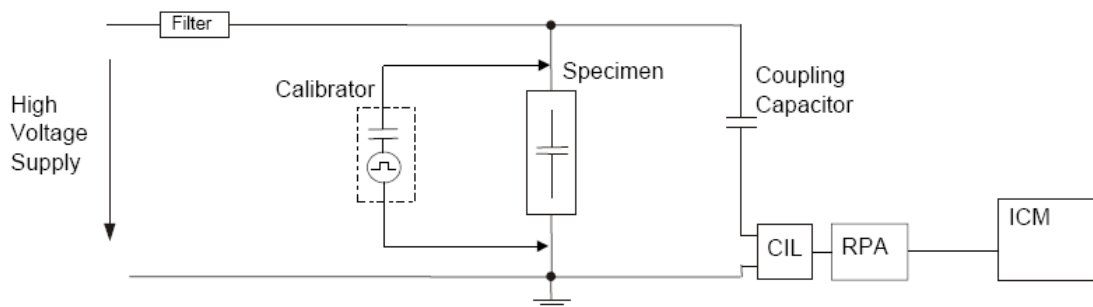
Figura 3. Esquema de conexiones para la calibración del sistema
