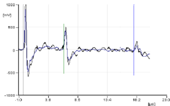
Reflectometría real de una señal de descargas parciales
