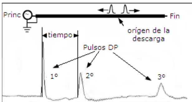
Reflectometría esquemática de una señal de descargas parciales
