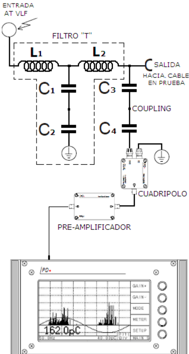
Esquema de medición de DP en el sistema VLF200-HVCD
