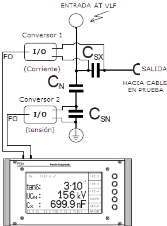
Esquema de medición de TD en el sistema VLF200-HVCD
