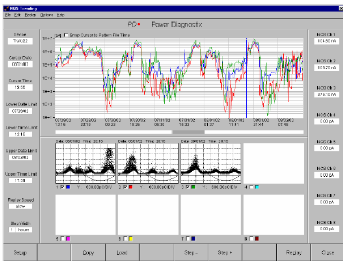
Fig.8, Registro de monitoreo continuo on-line sobre generador
