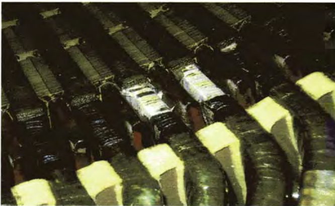
Fig.2, Defectos en la salida del slot en la aislación de un motor VPI.
