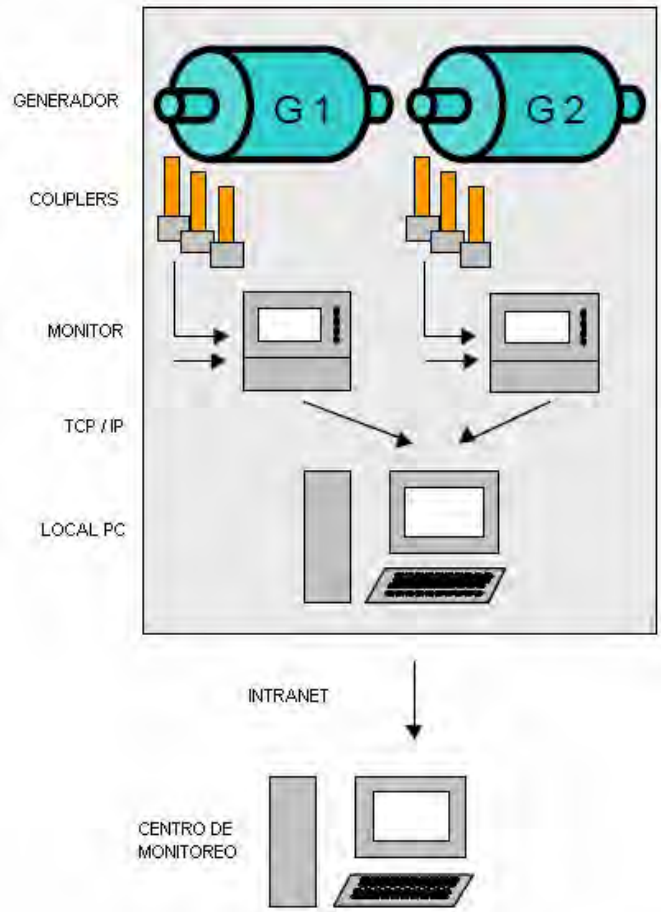
Fig 7 Diagrama de un sistema de monitoreo On-Line
