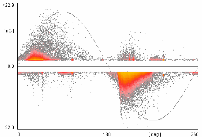
Fig.2, Defectos en la salida del slot en la aislación de un motor VPI.
