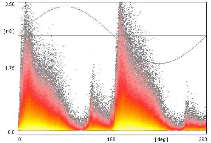
Fig. 3, Patrón PRPD: Aislación envejecida térmicamente.
