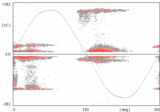
Fig. 6, Defecto en la salida del slot, etapa final, fuertes arcos.
